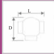
#206 Ball Tee
